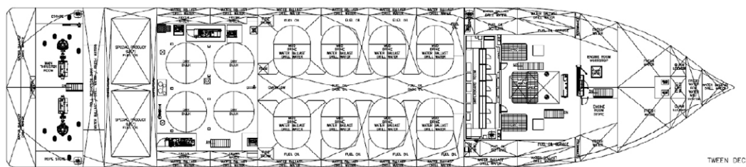
TWEEN DECK
